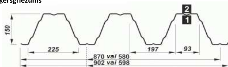
Šķērsgriezums
