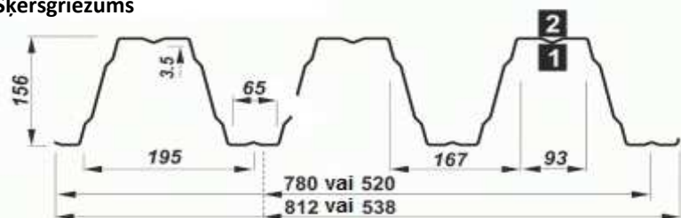
Šķērsriezums
