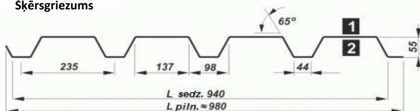
Šķērsriezums
