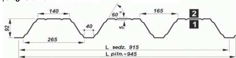
Šķērsriezums
